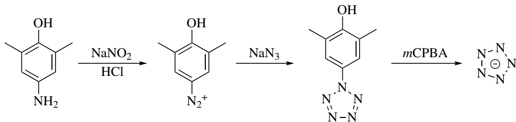
图 5: \text{N}_5^- 的合成路线及其结构
