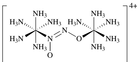
图 8: [\text{Co}_2(\text{NH}_3)_{10}(\text{N}_2\text{O}_2)]^{4+} 的结构
